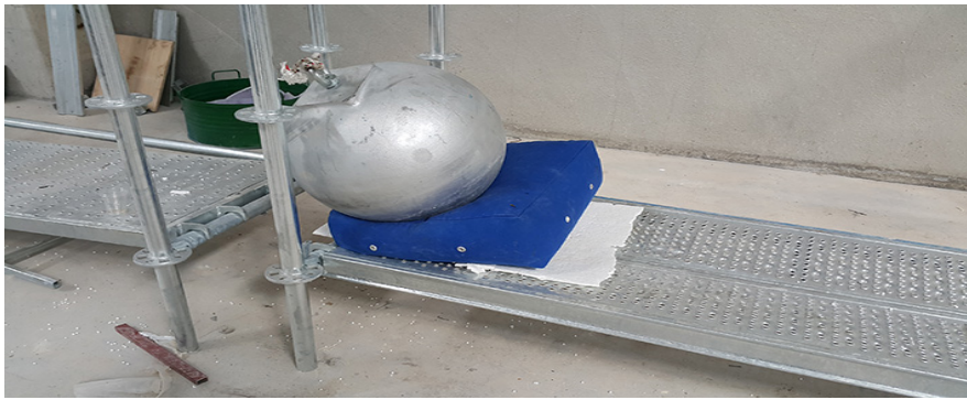
Şekil 2. Düşme deneyi
